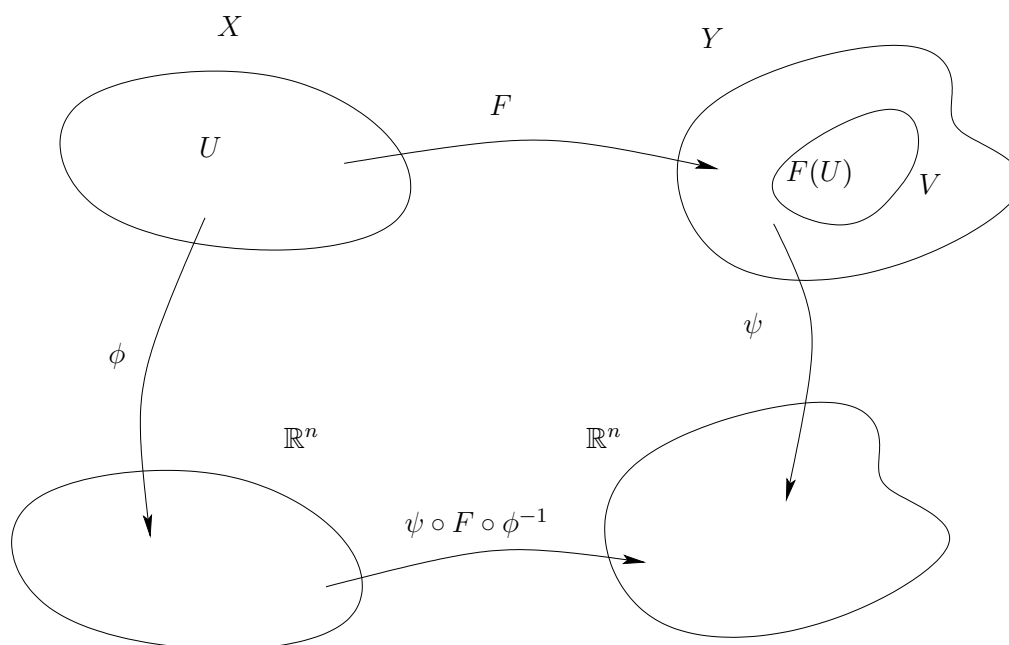
Kuva 2.1 — Differentioituva kuvaus.
