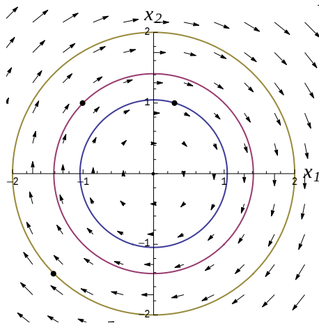
Kuva 4.1 — Tason vektorikentän V(x) = x^2 \frac{\partial}{\partial x^1} - x^1 \frac{\partial}{\partial x^2} integraalikäyriä. Esimerkin 3.11 nojalla vektorikentän V lauseke napakoordinaateissa on -\frac{\partial}{\partial \theta} .
