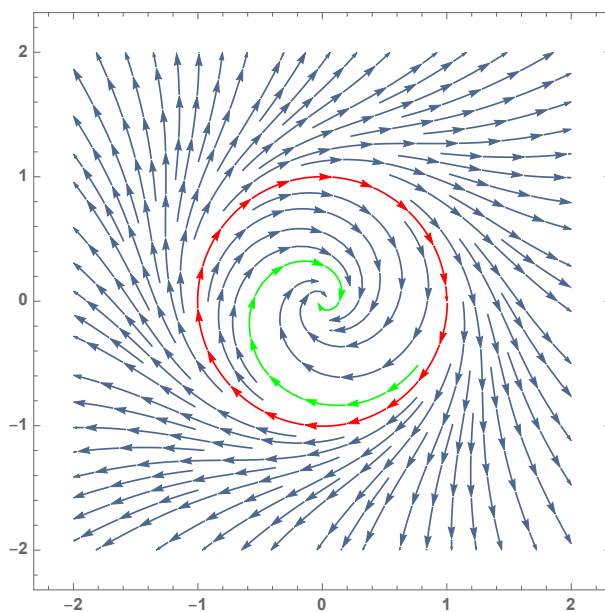
Kuva 4.2 — Napakoordinaateissa ilmoitetun tason vektorikentän \frac{r(r^2-1)}{2} \frac{\partial}{\partial r} - \frac{\partial}{\partial \theta} integraalikäyriä.
