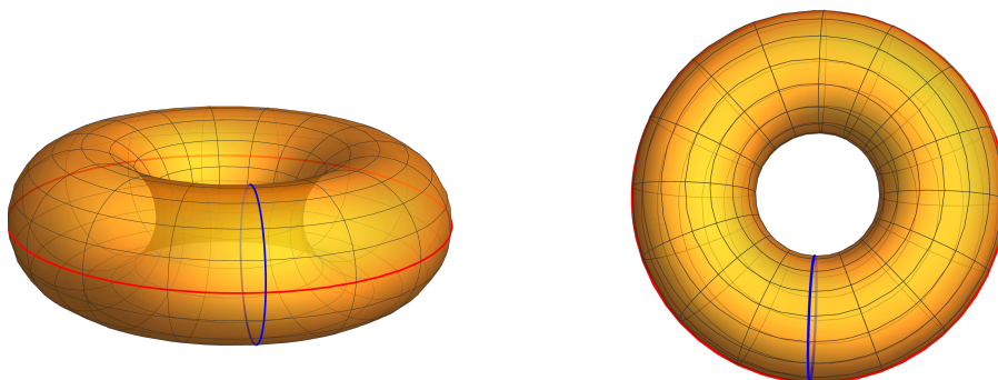
Kuva 1.5 — 2-torus.
