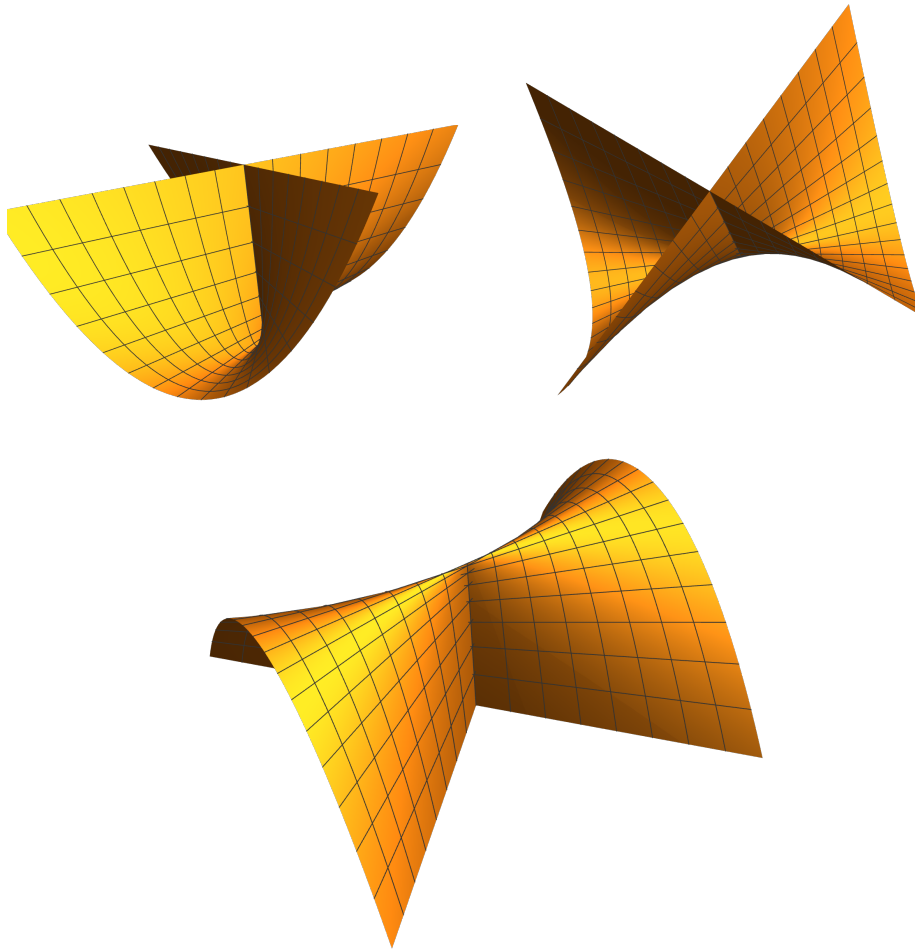
Kuva 5.2 — Whitney'n sateenvarjo kolmesta eri suunnasta.
