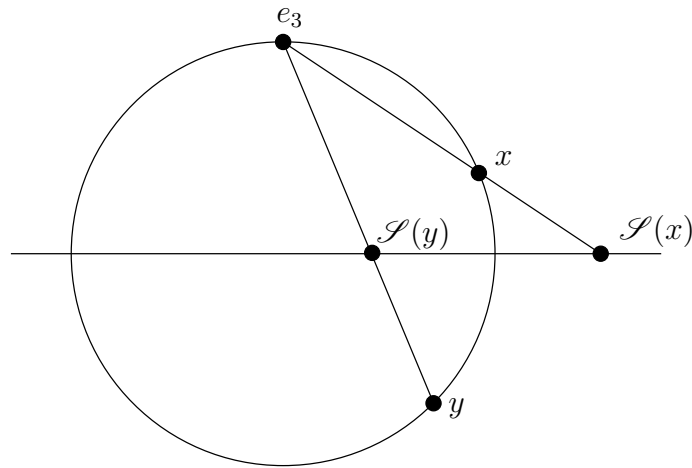
Kuva 1.2 — Stereograafinen projektio.
