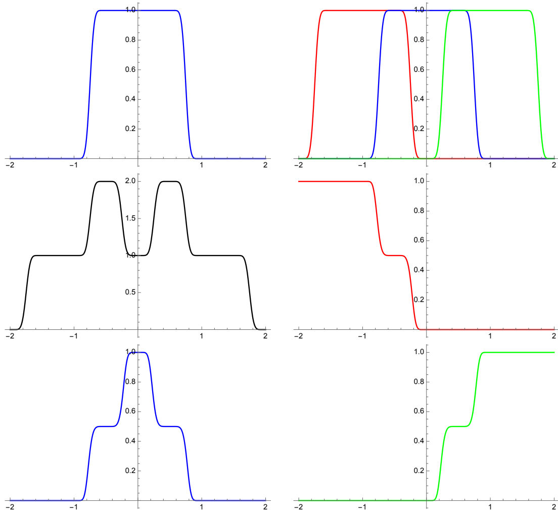
Kuva 10.1 — Ylimmällä rivillä vasemmalla tøyssyfunktio \rho_{-1,-\frac{1}{2},\frac{1}{2},1} ja oikealla kolme tøyssyfunktiota, joiden kantajat peittävät avoimen välin ] -2, 2[ . Toisella rivillä vasemmalla kolmen tøyssyfunktion summa ja sen jälkeen summafunktion skaalattujen tøyssyfunktioiden kuvaajat.
