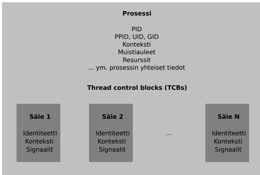
Kuva 24: Voidaan ajatella että säikeet (yksi tai useampia) sisältyvät prosessiin. Prosessi määrittelee koodin ja resurssit; säikeet määrittelevät yhden tai useampia rinnakkaisia suorituskohdita.
