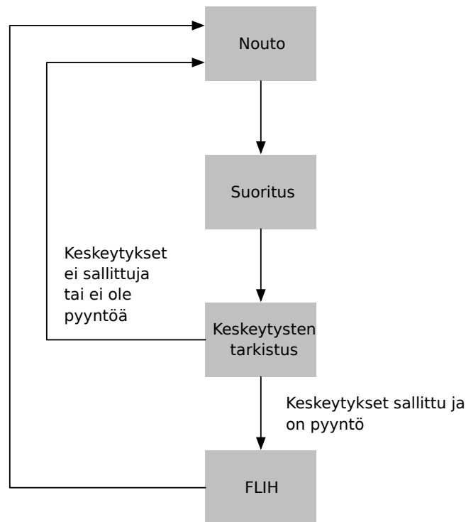
Kuva 19: Prosessorin suoritussykli: nouto, suoritus, tilan päivittyminen, mahdollinen keskeytyksen hoitoon siirtyminen.
