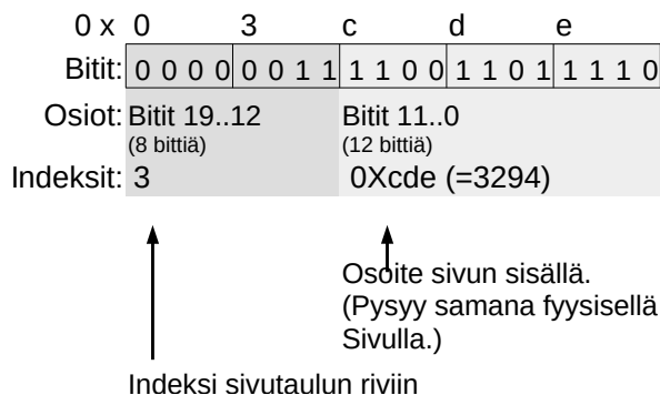
Kuva 28: Leikkiesimerkki prosessin virtuaalimuistiosoitteesta 20-bittisellä virtuaaliosoitteavaruudella ja 4096 tavun sivukoolla.
