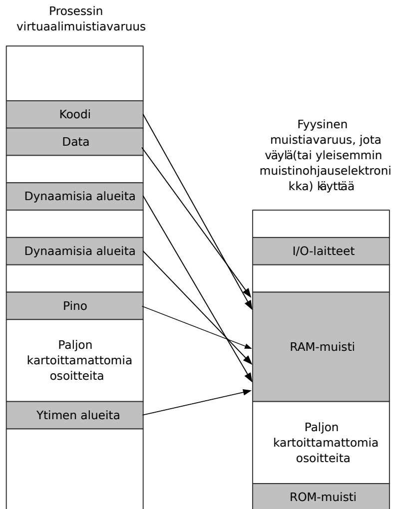
Kuva 16: Geneerinen esimerkki ohjelman näkemän virtuaaliosoiteavaruuden ja tietokonelaitteiston käsittelemän fyysisen osoiteavaruuden välisestä yhteydestä.
