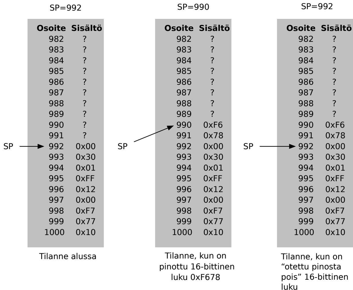
Kuva 12: Suorituspino: muistialue, jota voidaan käyttää push- ja pop-käskyillä. SP osoittaa aina pinoon "huippuun", joka "kasvaa" muistiosoitteen mielessä alaspäin.
