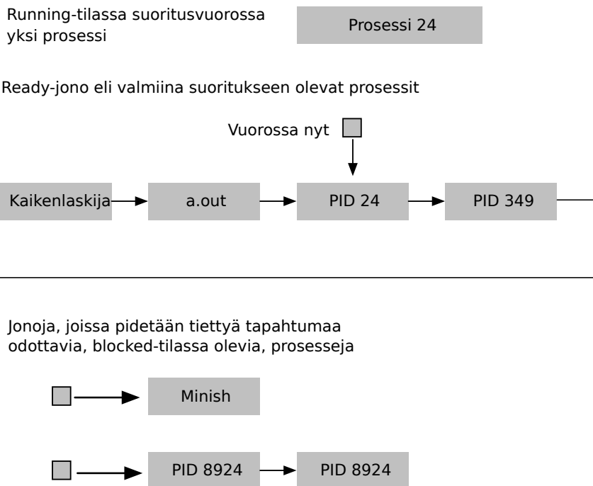
Kuva 22: Prosessien vuorontaminen kiertojonolla (round robin). Prosesseja siirretään kiertojonoon ja sieltä pois sen mukaan, täytyykö niiden jäädä odottelemaan jotakin tapahtumaa (eri jonoon, blocked-tilaan).
