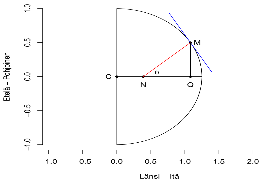
Kuva 1: Maan itäinen puolisko poikkileikkauksena akselin suhteen. Paikan M leveysaste on \phi .
